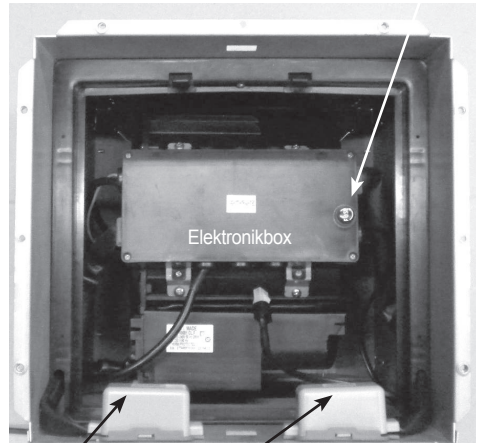
Anschlussbox Geruchssensor
